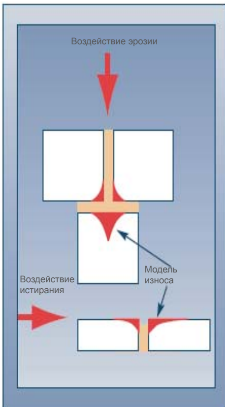
Широкие швы увеличивают истираемость и эрозию
